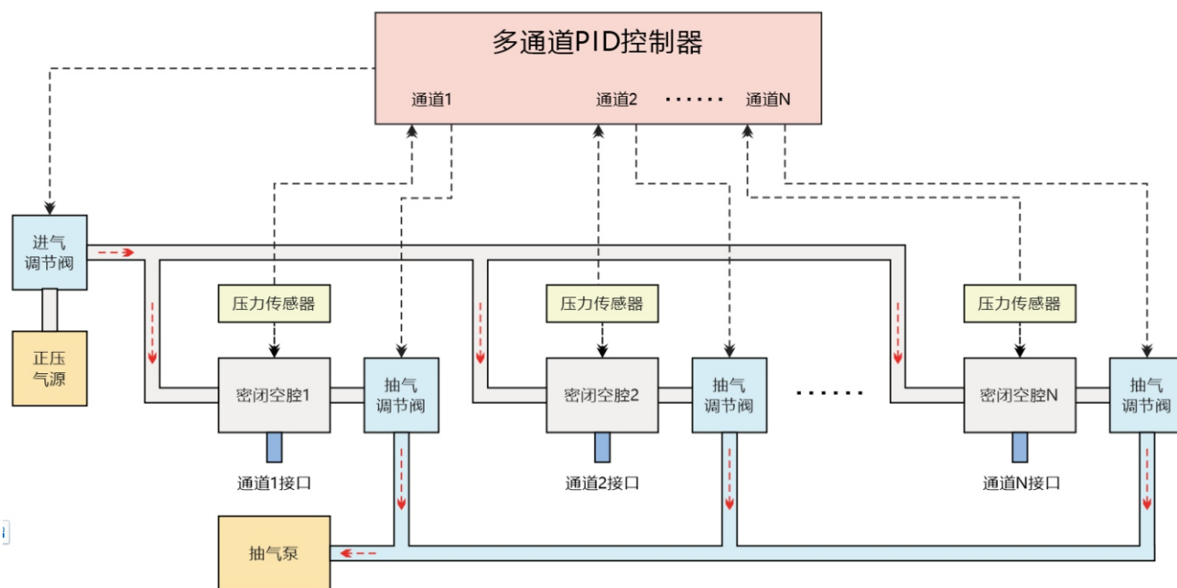
图2 微流控芯片进样用多通道压力控制器工作原理图
