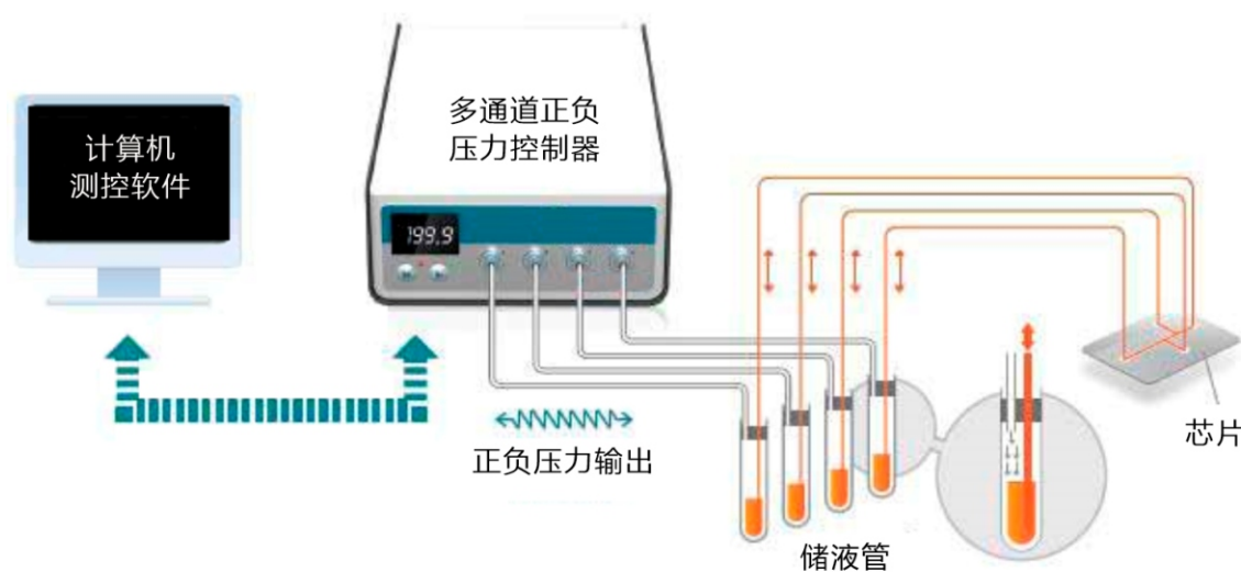
图1 多通道压力控制器在微流控芯片进样中的典型应用
