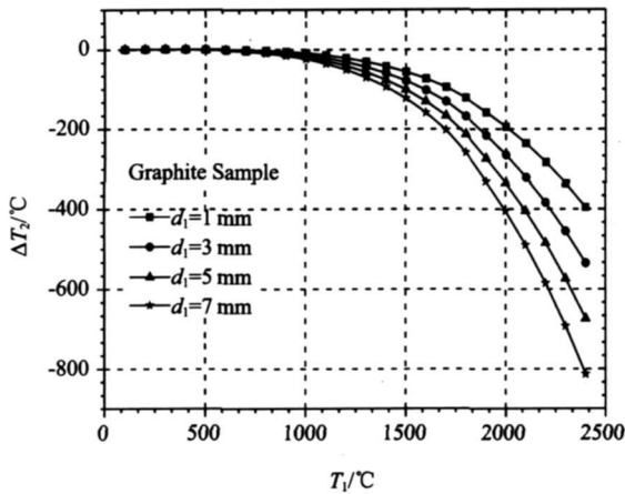
图8 石墨试样不同厚度温差测量结果
