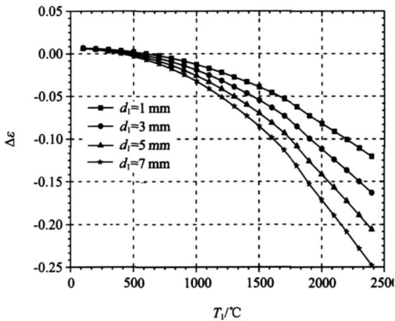
图9 发射率测量结果与试样厚度的关系
